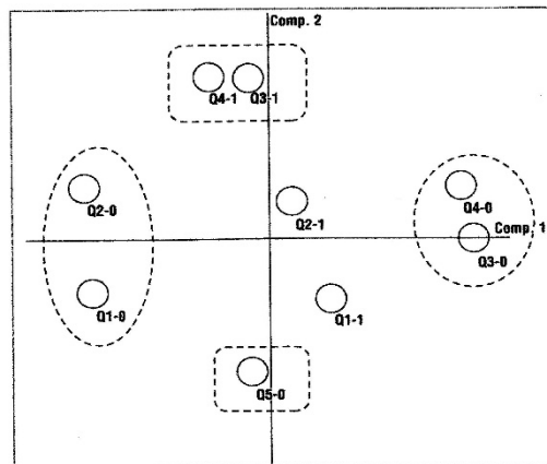
図2 構造行列(表2)の図示 第1主成分Comp.1と第2主成分Comp.2に 対する各共通数量化変数Qj-hの関係を表す
