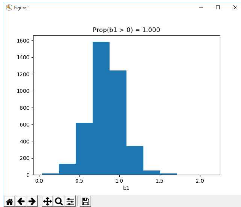
図 11.E.2.1 リスト 11.E.2.2 の実行時に表示されるグラフ
