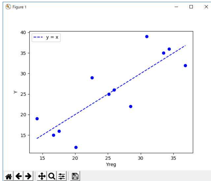
図 11.E.2.2 単回帰モデルによる予測値 Yreg とデータ値 Y の関係
